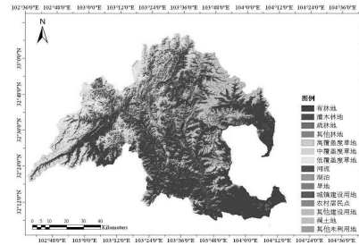
图 5 2010 年地表覆盖分类图
