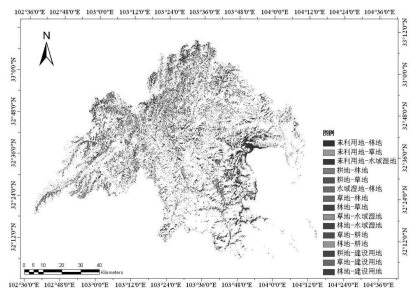
图 6 2000-2010 年地表覆盖变化图
