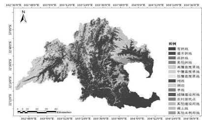
图 4 2000 年地表覆盖分类图
