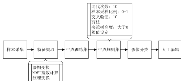
图 3 基于决策树算法的分类步骤
