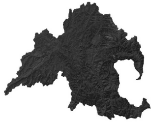
图 2 2010 年预处理后松潘县 Landsat-5 TM 影像
